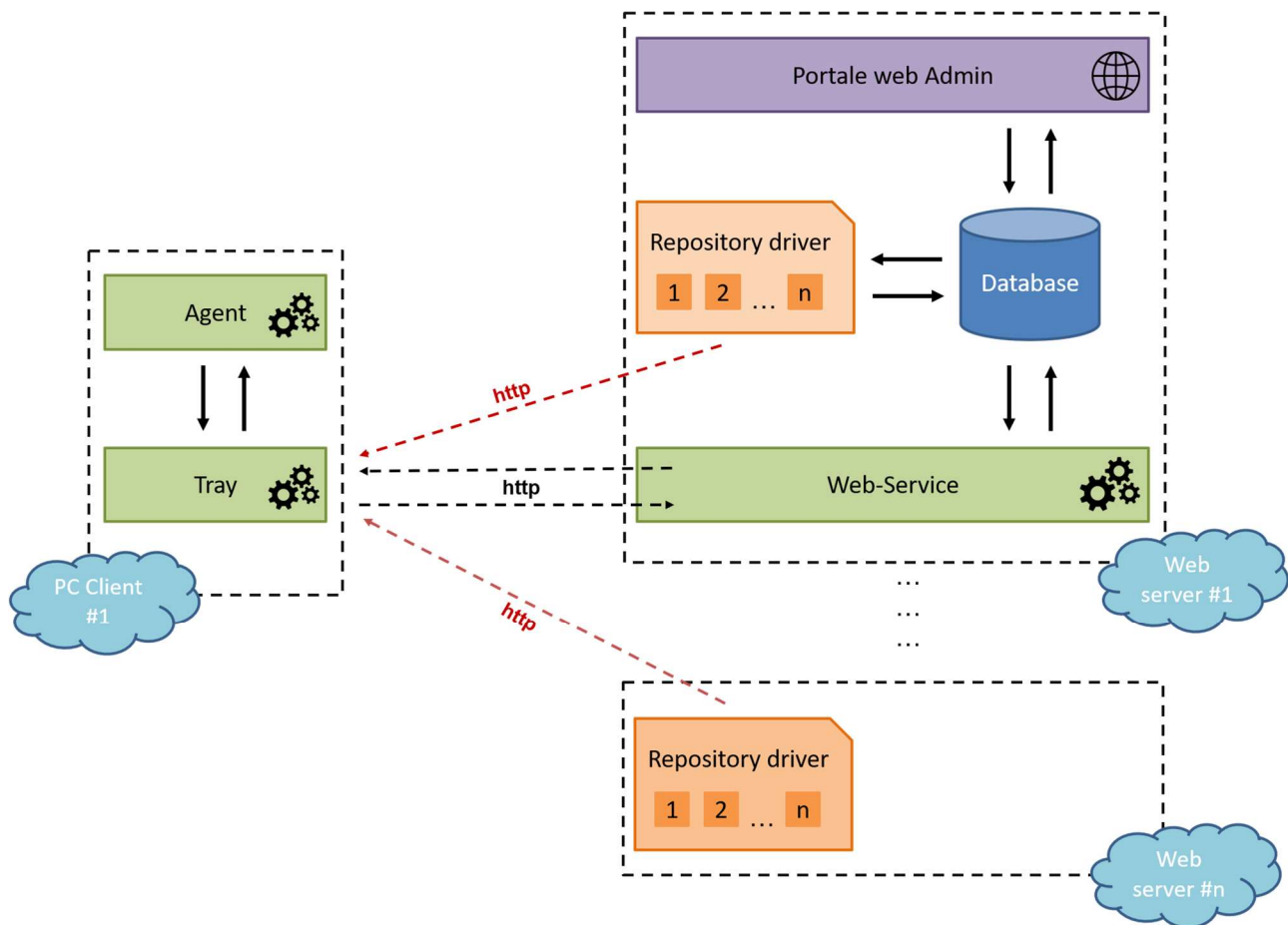
Gest-Q - Architettura della soluzione
